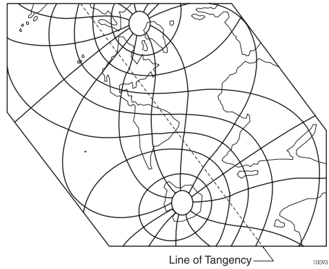
Figure 4.4. Oblique Mercator
