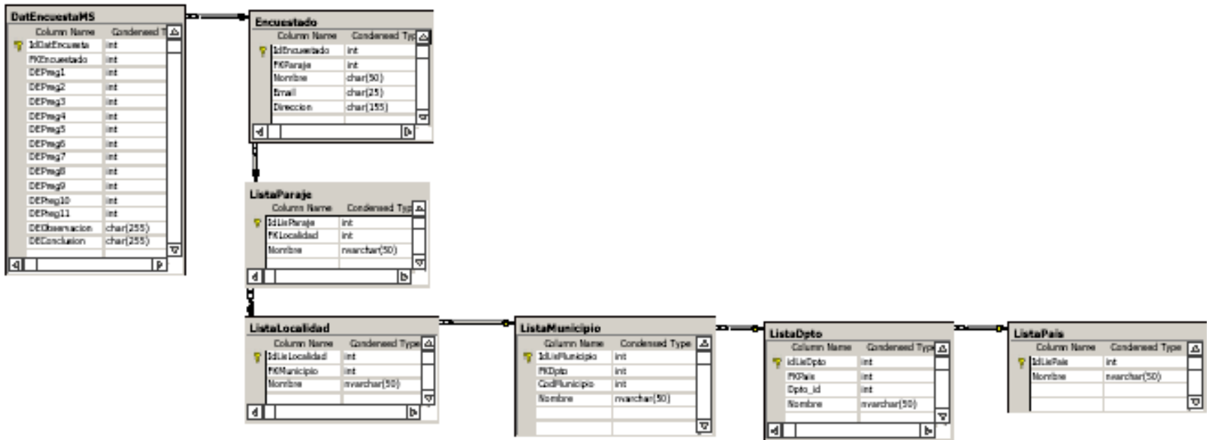
Diagrama Entidad Relación de Encuestas MacroSísmicas
