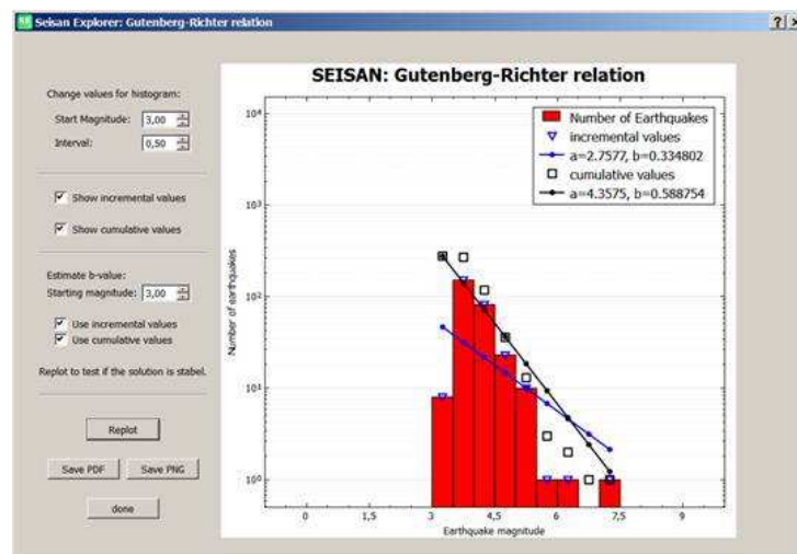
Figure 4.7: se-gutenberg-richter
