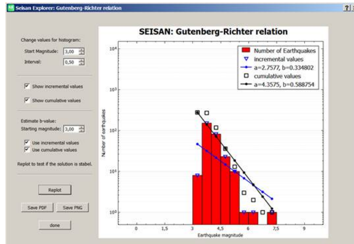
Figure 4.7: se-gutenberg-richter
